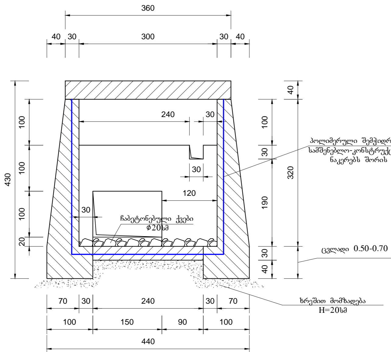
ტიპური კრილი კაშხლის ტანში
