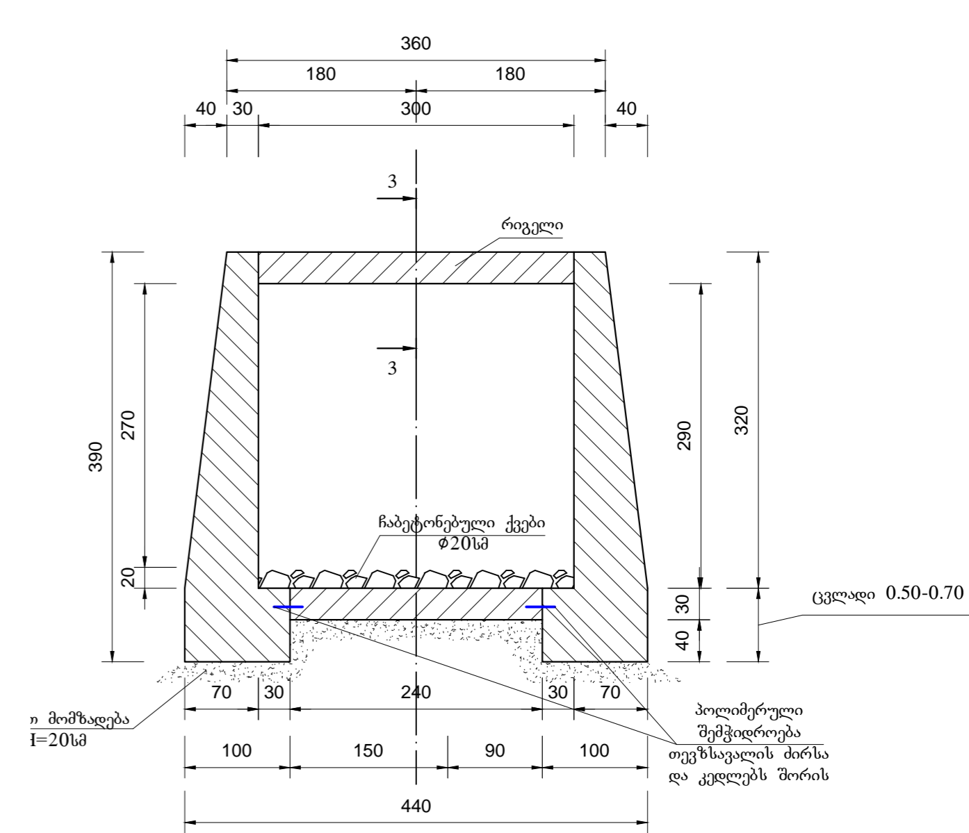
ტიპური კრილი 2-2
