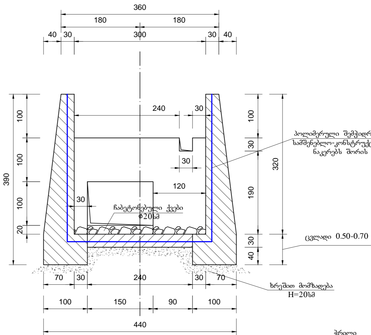
ტიპური კრილი 1-1
