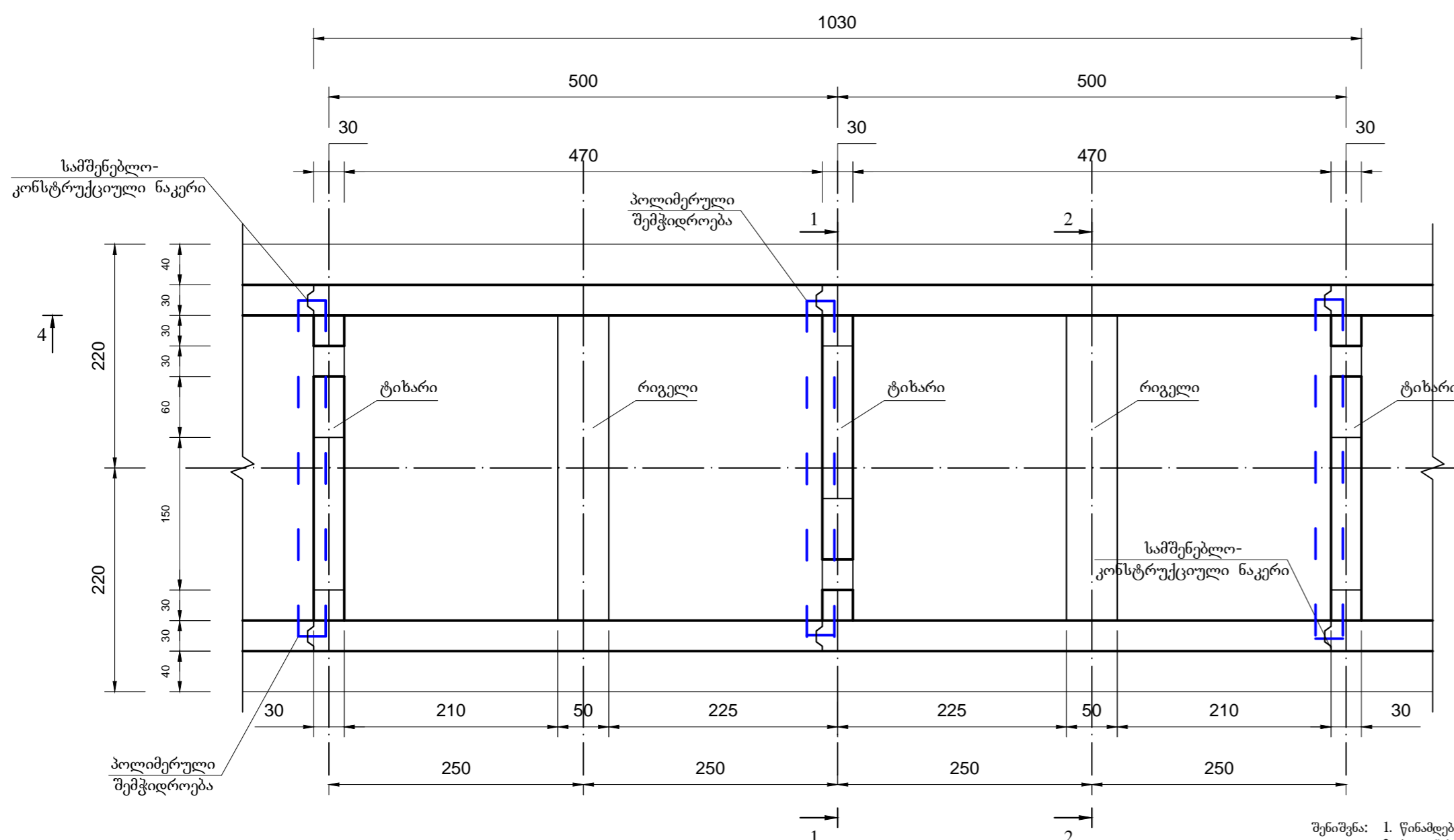
გრძივი კრილი
