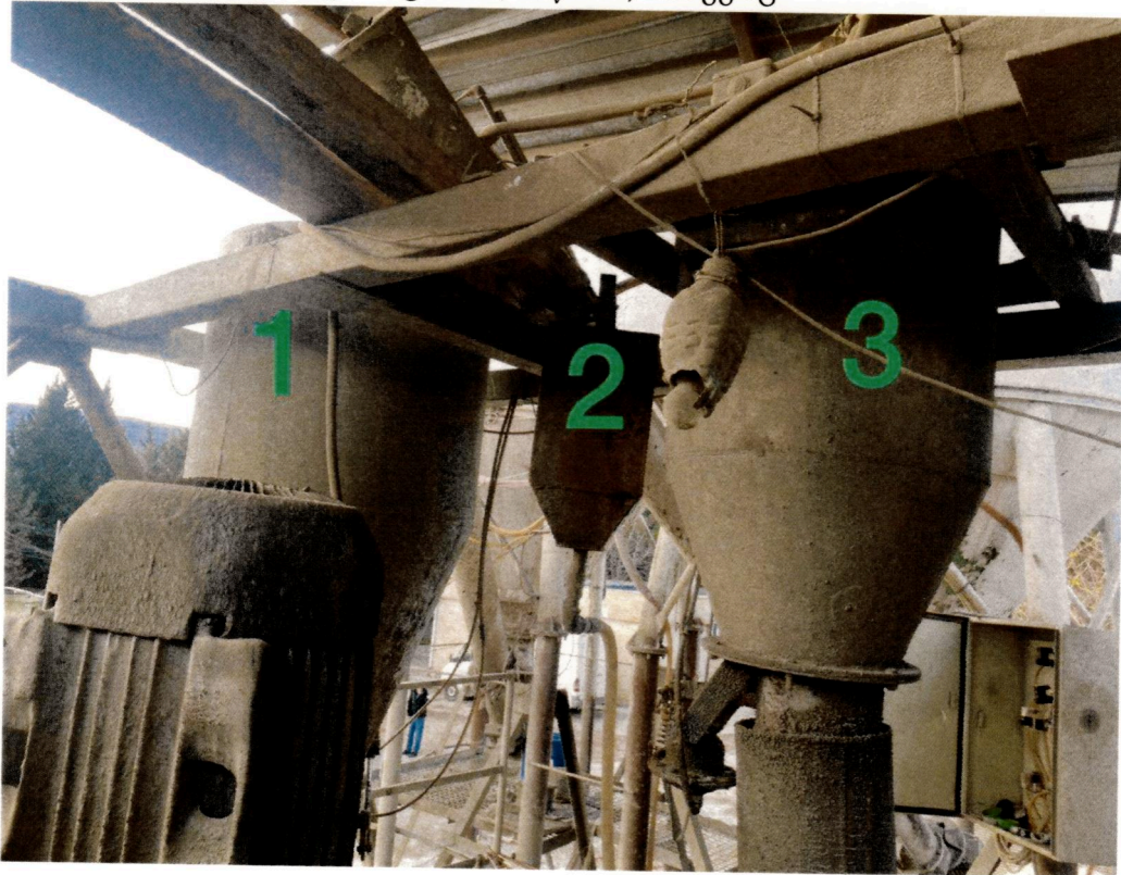
ბეტონის ამრევი SB-138. მოცულობა 1.5მ 3 (ძრავი 37კვტ/940 ბრნ.წუთი) 1ცალი
