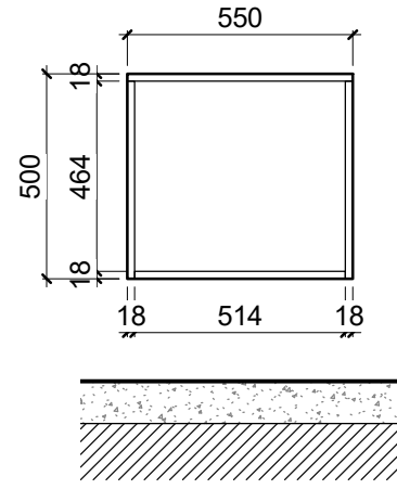
BLF-31 - გვერდხედი 1 : 20 BLF-30, BLF-31 - სათავსი
