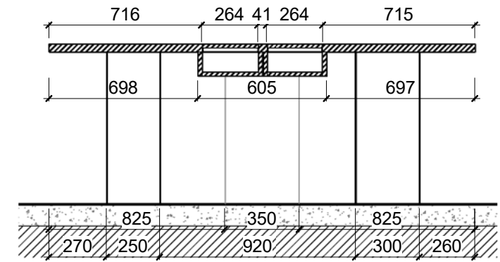
BLF-28 - გან. კრილი 1 : 25 BLF - 28 - მაგიდა
