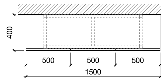
BLF-29 - ზედხედი 1:25 BLF-25-3, BLF-29 - სათავსი
