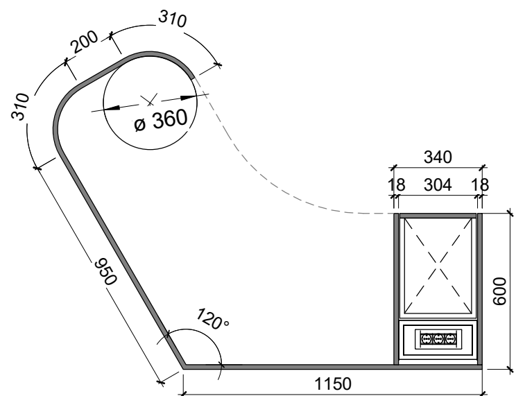
BLF-06 - კორ. კრილი 1 : 20 BLF-06 - მიმღების მაგიდა
