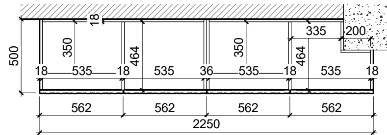
BLF-25-3 - წინხედი 1:25 BLF-25-3, BLF-29 - სათავსი
