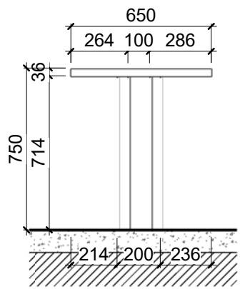
BLF-27-B-1,2 - გვერდხედი BLF-27-A-1,2,3 27-B-1,2 - მაგიდა
