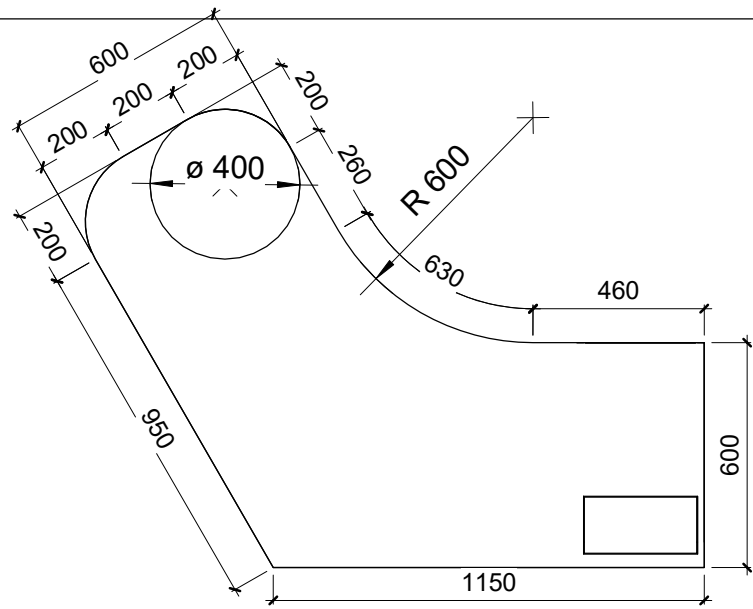
BLF-06 - ზედხედი 1 : 20 BLF-06 - მიმღების მაგიდა
