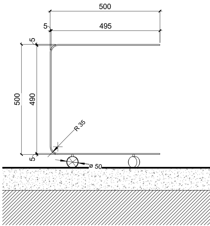
BLF-08-A - გვერდხედი 1 : 10 BLF-08-A
