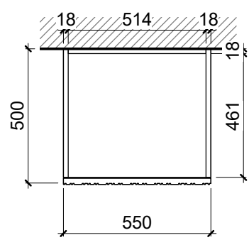
BLF-31 - ჰორ. კრილი 1 : 20 BLF-30, BLF-31 - სათავსი
