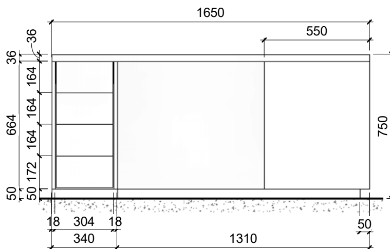
BLF-06 - ხედი 1 1 : 20 BLF-06 - მიმღების მაგიდა
