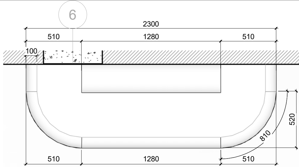
BLF-09 - ზედბედი 1 : 20 BLF - 09, BLF - 20, რბილი ავეჯი
