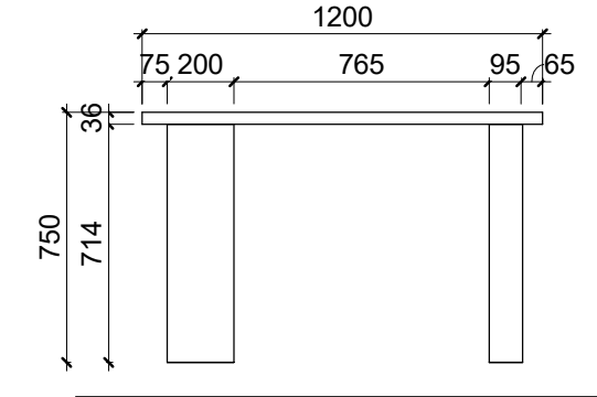
BLF-27-B-1,2 - ჰორ. კრილი BLF-27-A-1,2,3 27-B-1,2 - მაგიდა
