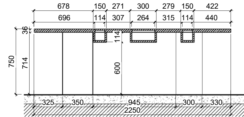
BLF-28 - გრძ. კრილი 1 : 25 BLF - 28 - მაგიდა
