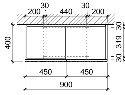
BLF-30 - ჰორ. კრილი 1 : 25 BLF-30, BLF-31 - სათავსი
