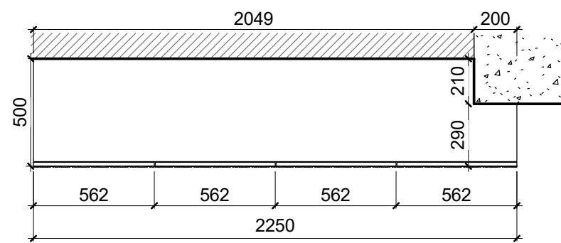
BLF-25-3 - ზედხედი 1:25 BLF-25-3, BLF-29 - სათავსი
