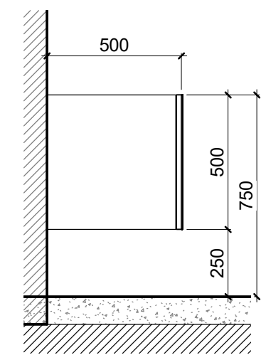
BLF-31 - გვერდხედი 1 : 20 BLF-30, BLF-31 - სათავსი
