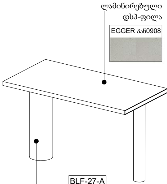
BLF-27-A-1,2,3 - გრძ. კრილი BLF-27-A-1,2,3 27-B-1,2 - მაგიდა
