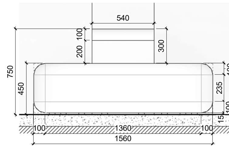
BLF-20 - წინხედი 1 : 20 BLF - 09, BLF - 20, რბილი ავეჯი
