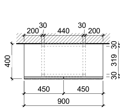
BLF-30 - ზედხედი 1 : 25 BLF-30, BLF-31 - სათავსი
