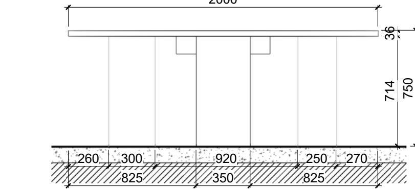
BLF-28 - წინხედი 1 : 25 BLF - 28 - მაგიდა
