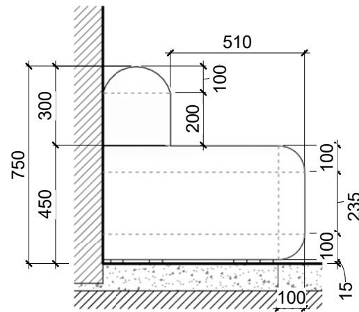
BLF-09 - გვერდხედი 1 : 20 BLF - 09, BLF - 20, რბილი ავეჯი
