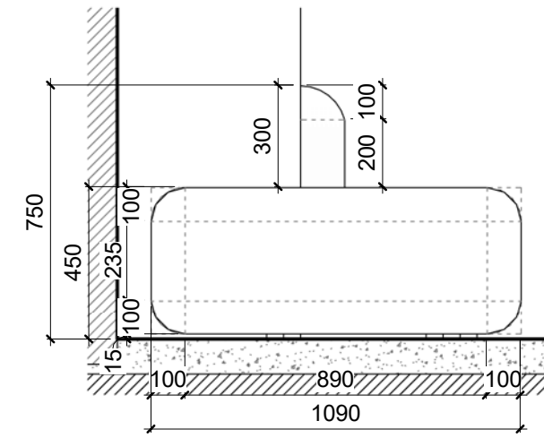
BLF-20 - გვერდხედი 1 : 20 BLF - 09, BLF - 20, რბილი ავეჯი
