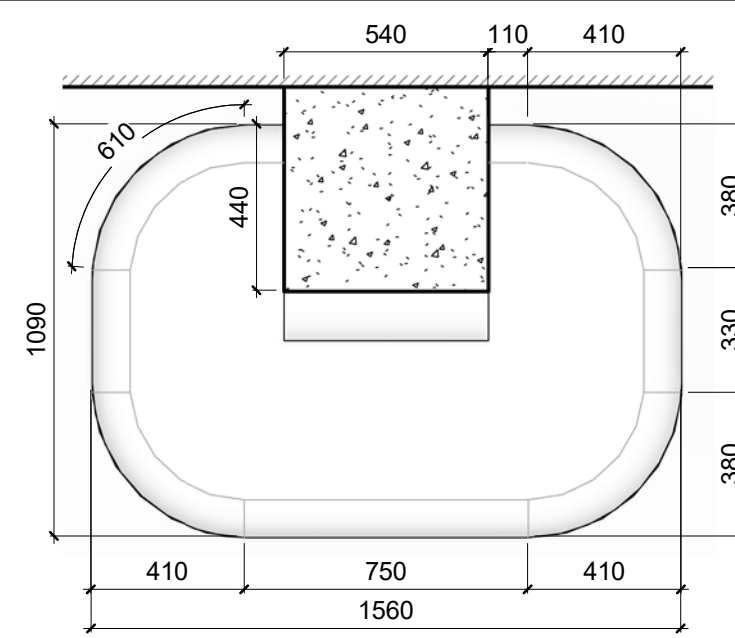
BLF-20 - ზედბედი 1 : 20 BLF - 09, BLF - 20, რბილი ავეჯი
