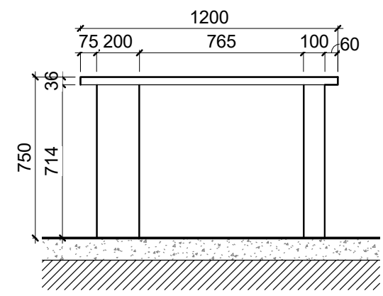
BLF-27-B-1,2 - გრძ. კრილი BLF-27-A-1,2,3 27-B-1,2 - მაგიდა
