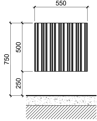
BLF-31 - წინხედი 1 : 20 BLF-30, BLF-31 - სათავსი
