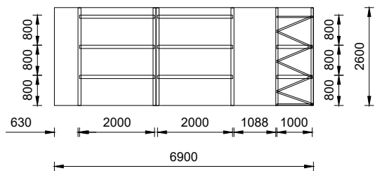
ჭრილი 2-2
