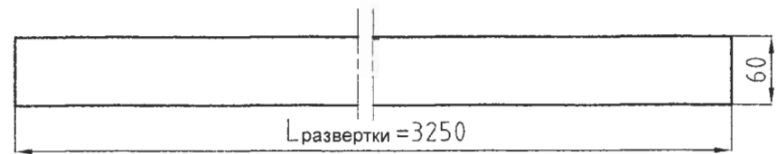
Дет. поз. 4
