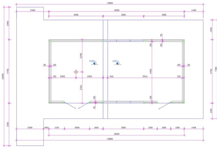
#134 ჭაბურღილის საკაპტაჟე ნაგებობა
