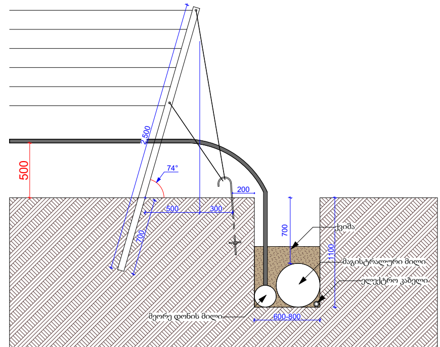
კვანძი 1 თავბოძისა და ორმოს მოწყობის ნახაზი ვარიანტი 2 (წვეთოვანის მილი 500 მმ სიმაღლეზე)
