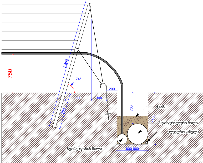
კვანძი 1 თავბოძისა და ორმოს მოწყობის ნახაზი ვარიანტი 1 (წვეთოვანის მილი 750 მმ სიმაღლეზე)
